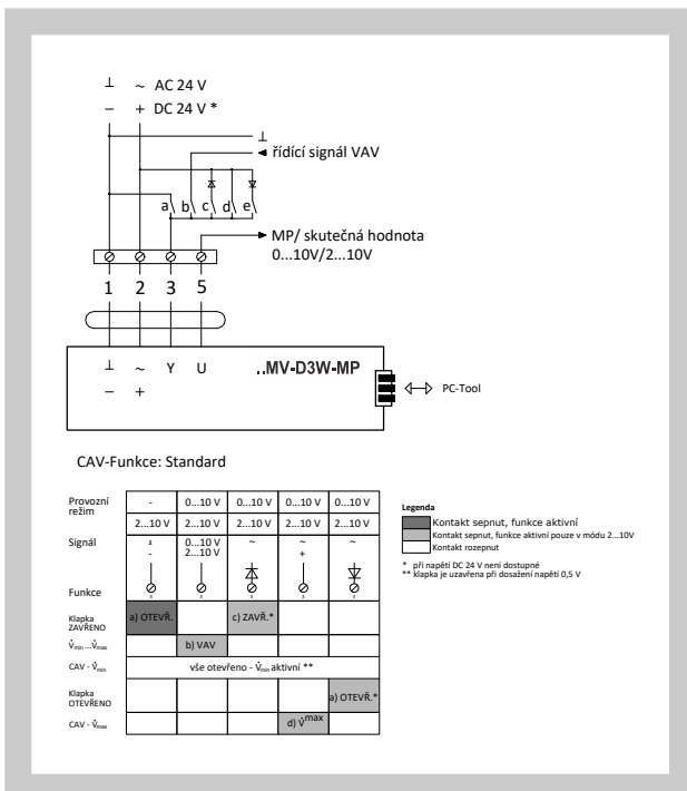
Obr. 11 Regulace průtoku vzduchu pomocí pohonu LMV-D3W-MP.1 MDK
