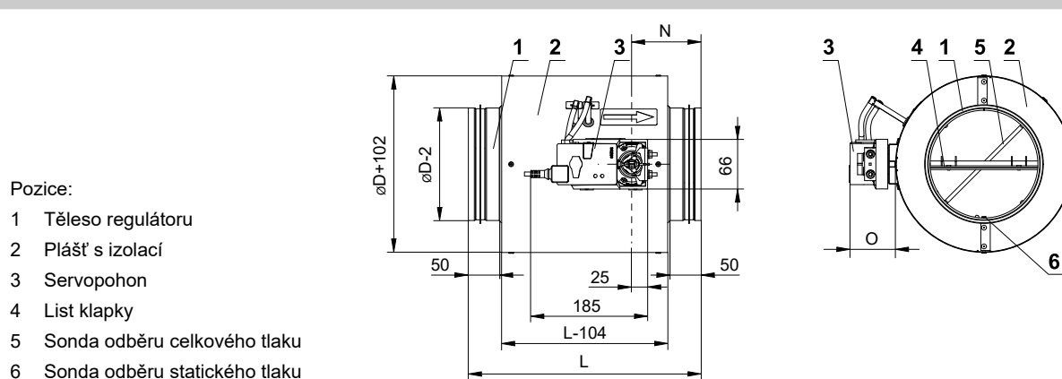
Obr. 5 RPM-LV s izolací
