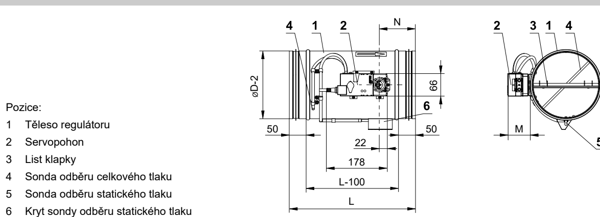
Obr. 5 RPM-LV s izolací
