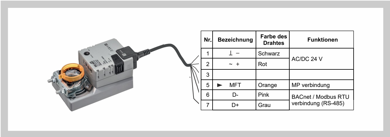
Abb. 13 Kompaktregler BELIMO LMV-D3W-MOD.1 MDK
