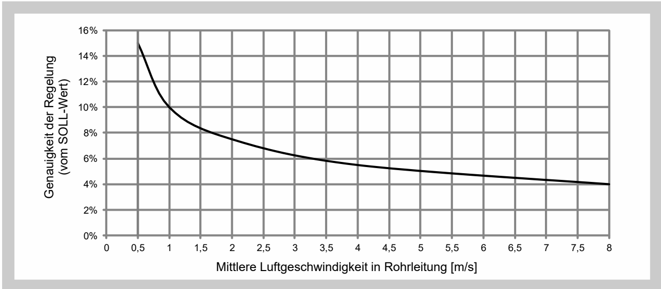
Diag. 1 Genauigkeit der Regelung für den Regelungsdruckverlust im Bereich von 10 Pa bis 600 Pa
