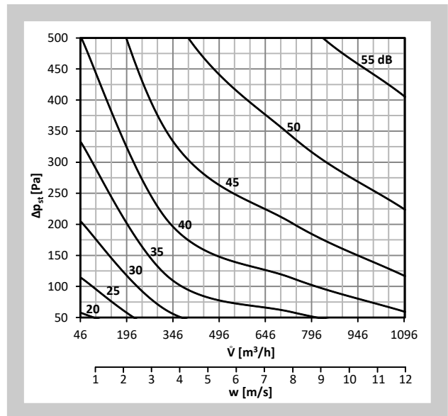
Diag. 19 Niveau der akustischen Leistung L_{wa} [dB(A)] ausgestrahlt außerhalb der Rohrleitung DN180, ohne Isolierung
